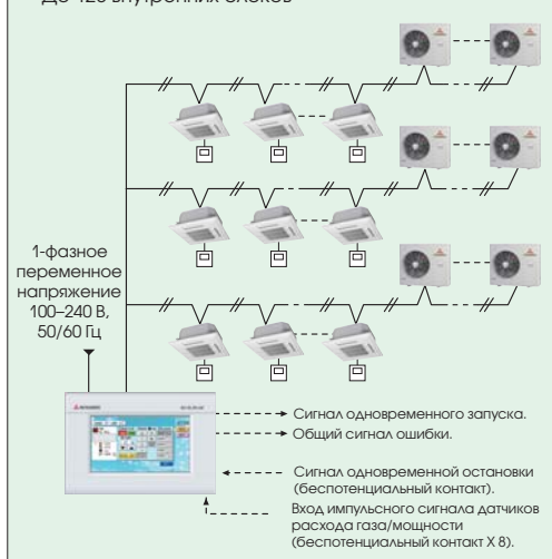
Схема сети
